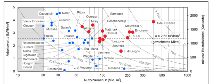
Nutzvolumen, Arbeitswerte und Energieinhalte der bestehenden grösseren Stauseen (> 20 Mio. m 3 ) in der Schweiz (Quelle: Felix et al., 2020).
